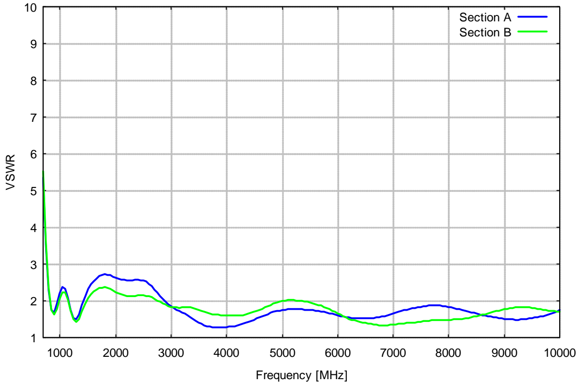
Stehwellenverhältnis
