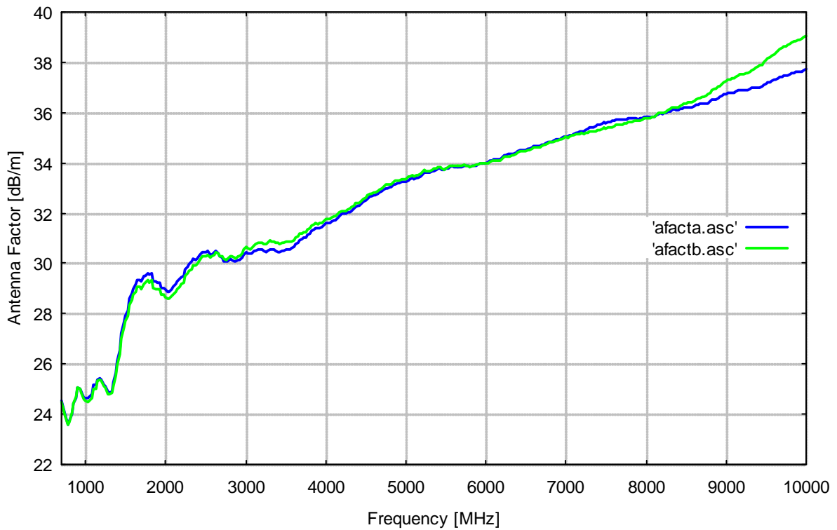
Antennenwandlungsmaß
